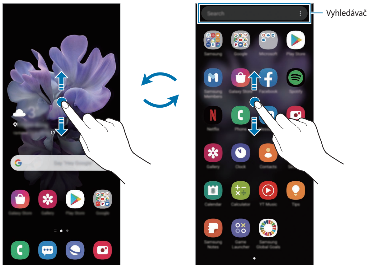
Domovská obrazovka
